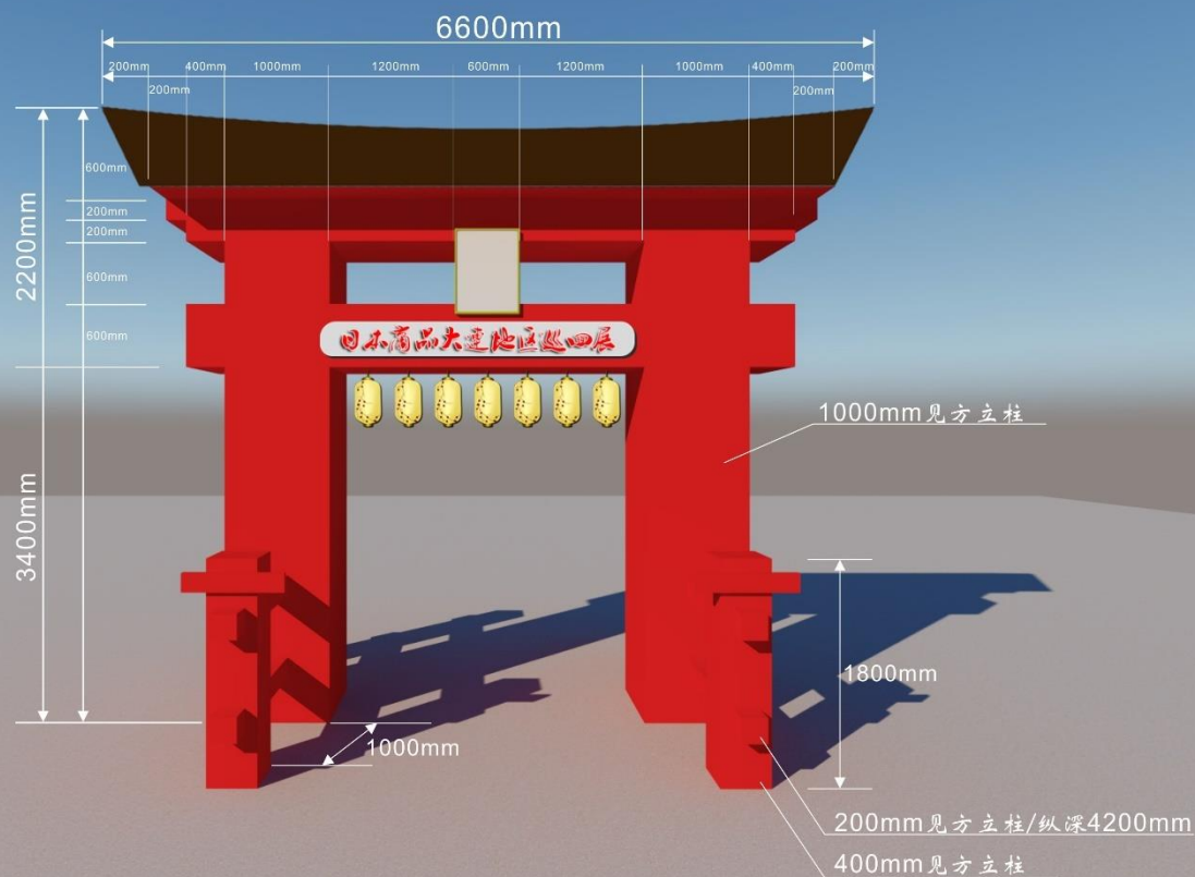
日本商品大連地区巡回展造型尺寸图
